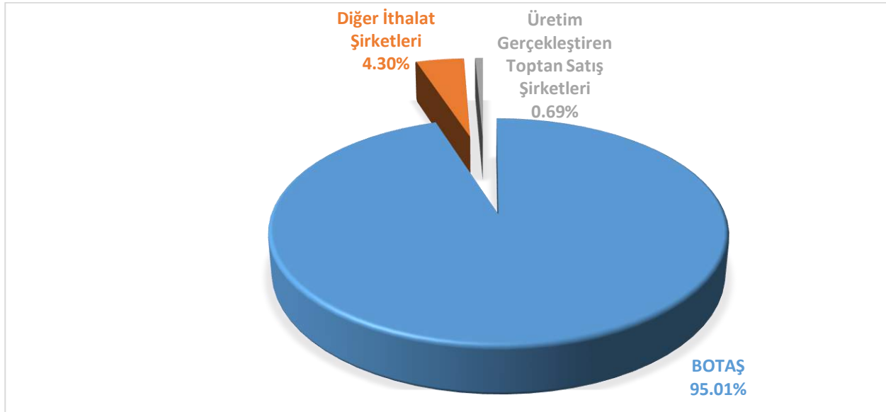
Şekil 4.1: 2022 Yılı İthalatçı Şirketler ve Üretim Şirketlerinin Doğal Gaz Arzındaki Payları(%)
