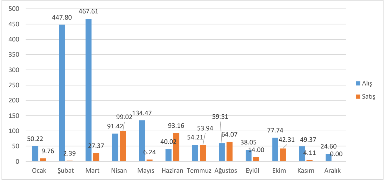
Şekil 4.2 2022 yılı aylara göre BOTAS tarafından Organize Toptan Satış Piyasasında Gerçekleştirilen İlave Dengeleyici Gaz Miktarı (Milyon Sm³)
