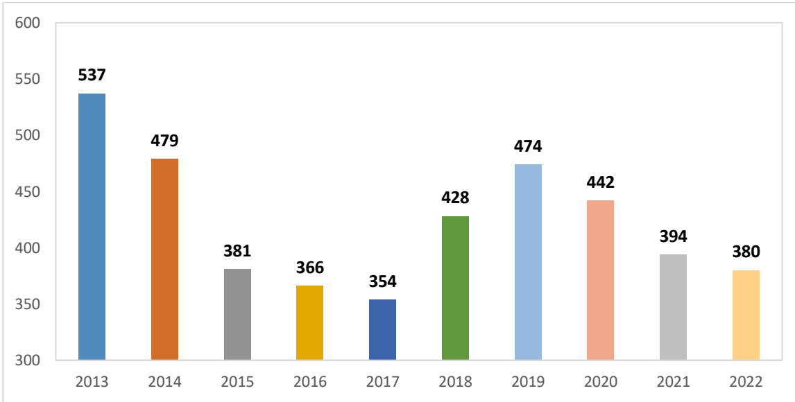
Şekil 1.1: 2012-2022 Yılları Doğal Gaz Üretim Miktarları (Milyon Sm 3 )
