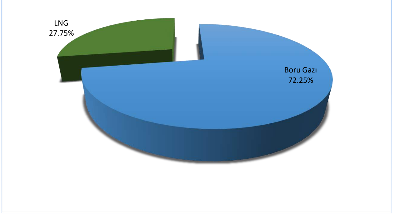
Şekil 2.5: 2022 Yılı Toplam İthalatta Boru Gazı-LNG Payları(%)
