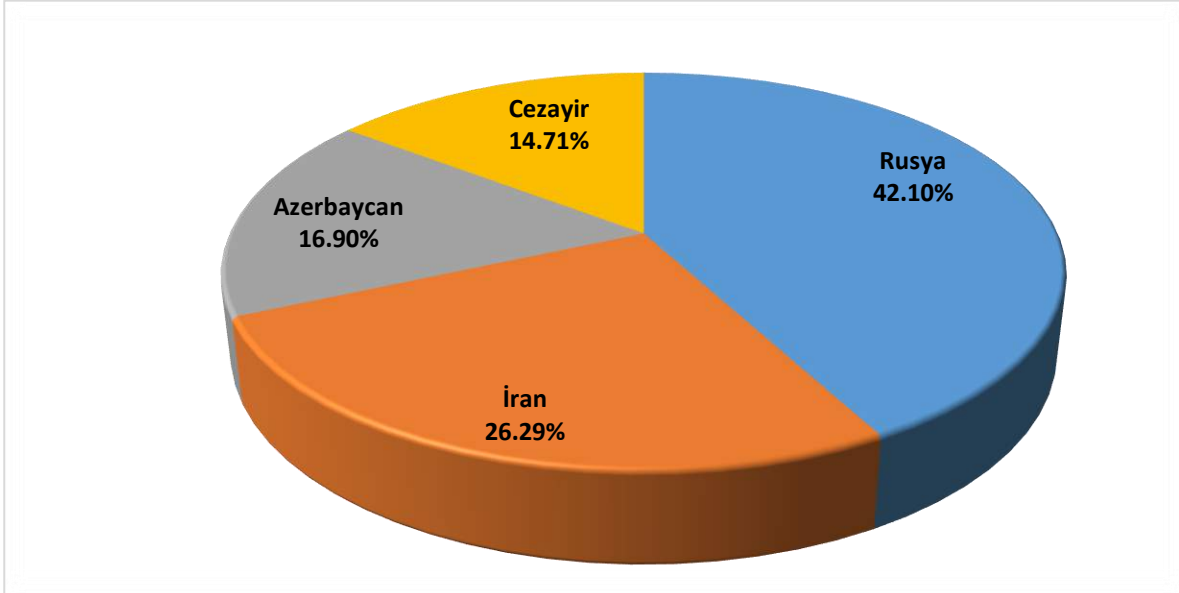
Şekil 2.7: 2022 Yılı Uzun Dönemli İthalat Lisansı Sahibi Şirketlerin İthalat Miktarlarının İthalatın Gerçekleştiği Ülkelere Göre Dağılımı(%)
