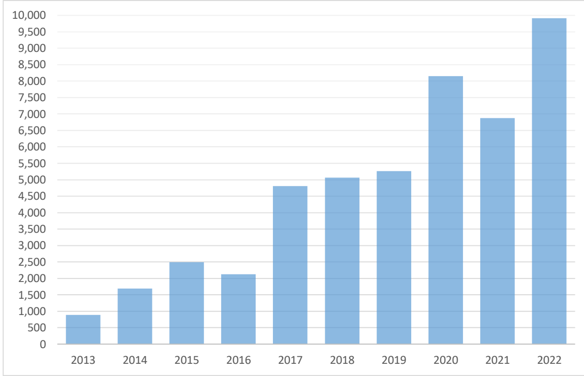
Şekil 2.11: 2013-2022 Yılları Arası Spot LNG İthalatı Değişimi (Milyon Sm³)
