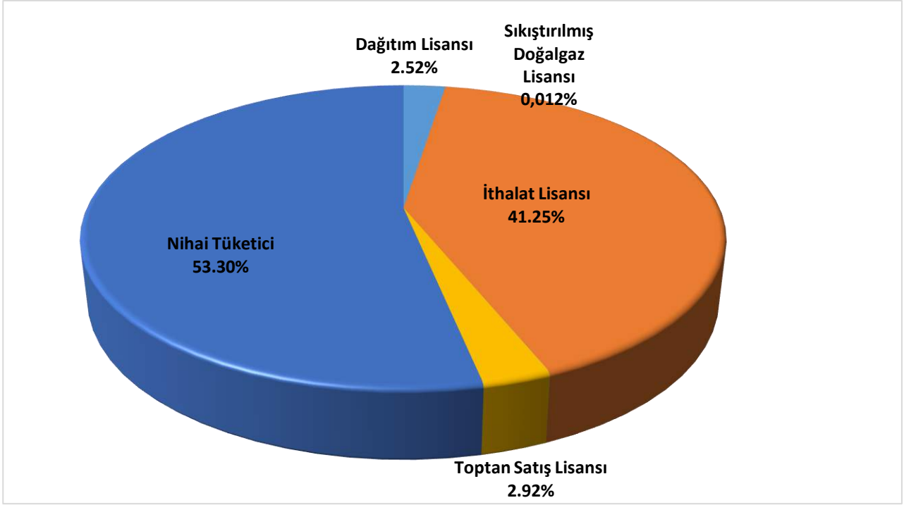
Şekil 1.6: 2022 Yılı Üretim Yapan Toptan Satış Lisansı Sahibi Şirketlerin Satış Yaptıkları Müşterilerin Payları(%)
