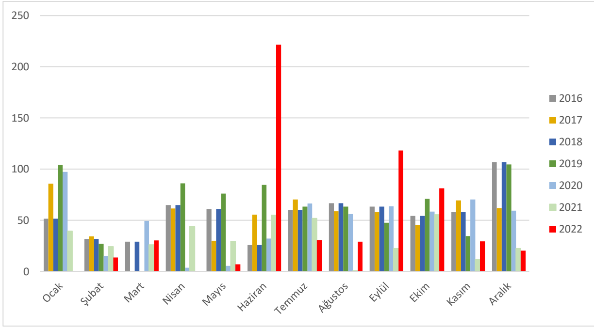
Şekil 2.15: 2016 ve 2022 Yılları Arasında İhraç Edilen Gaz Miktarının Aylara Göre Karşılaştırması (Milyon Sm³)
