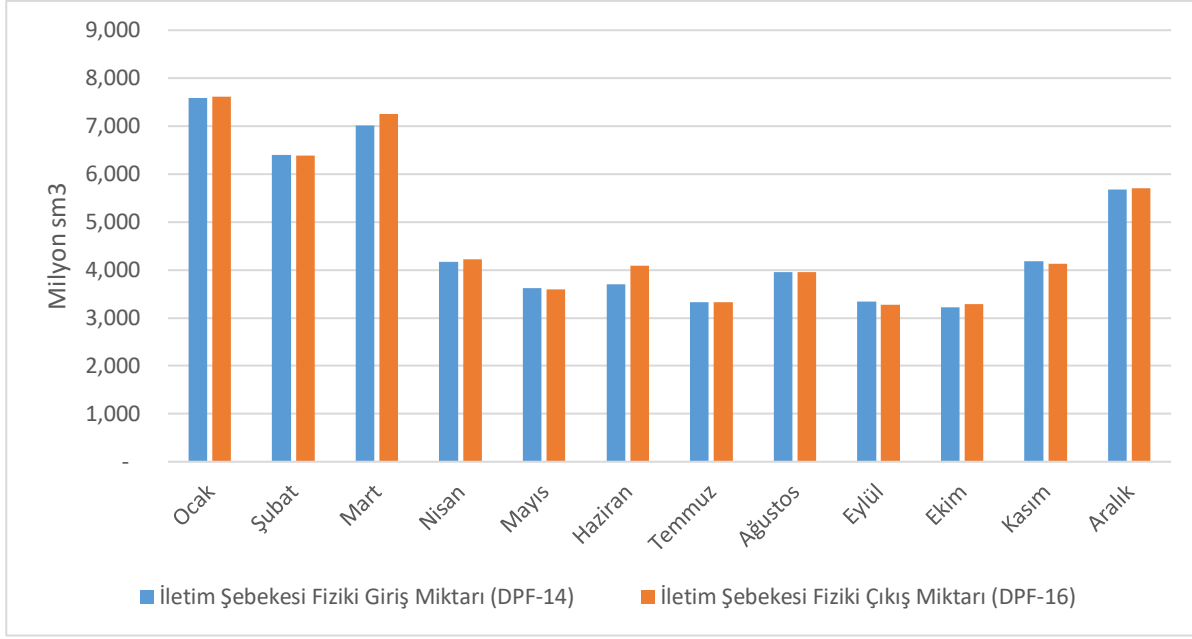
Şekil 6.1: 2022 Yılında İletim Şebekesine Giriş ve Çıkış Yapan Doğal Gaz Miktarının Aylık Dağılımı (Milyon Sm³)
