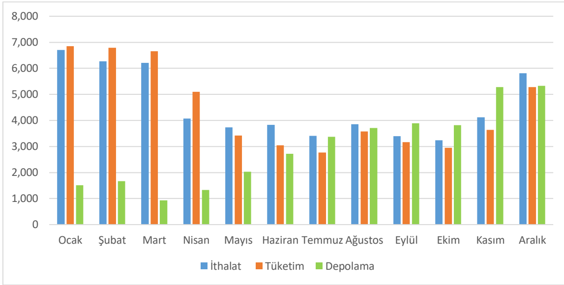
Şekil 3.2: 2022 Yılında Aylara Göre İthalat-Tüketim-Stok Miktarları Karşılaştırması (Milyon Sm³)
