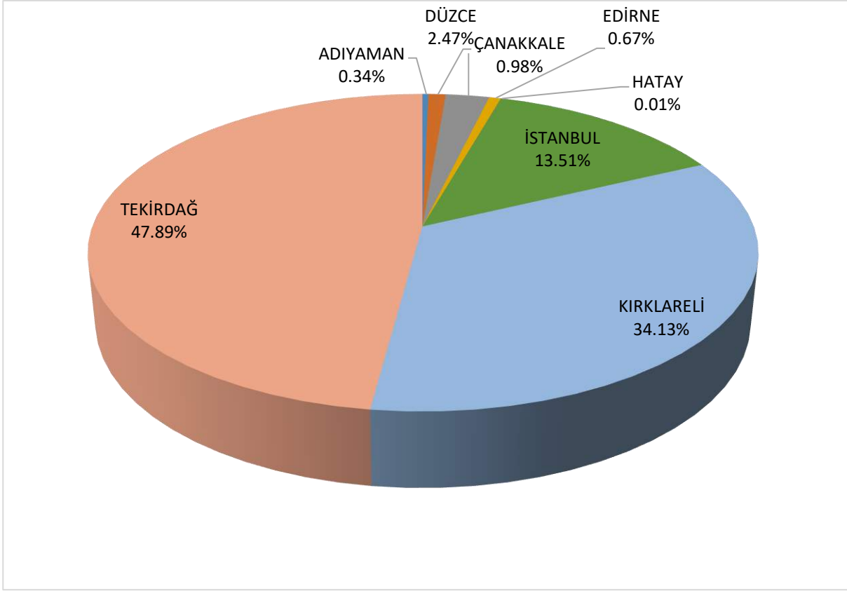
Şekil 1.3: 2022 Yılı Üretim Sahalarının Bulunduğu İllere Göre Doğal Gaz Üretim Oranları(%)
