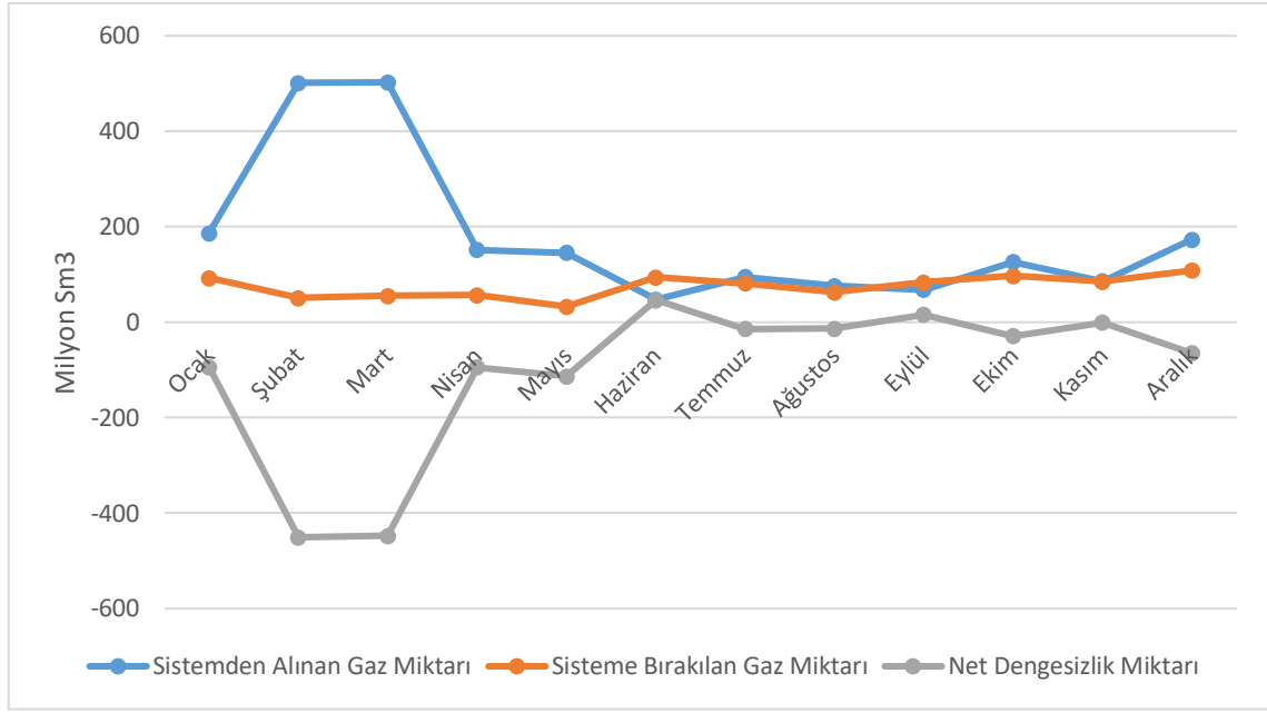
Şekil 6.4: 2022 Yılında İletim Şebekesinde Gerçekleşen Dengesizlik Miktarının Aylık Dağılımı (Milyon Sm³)
